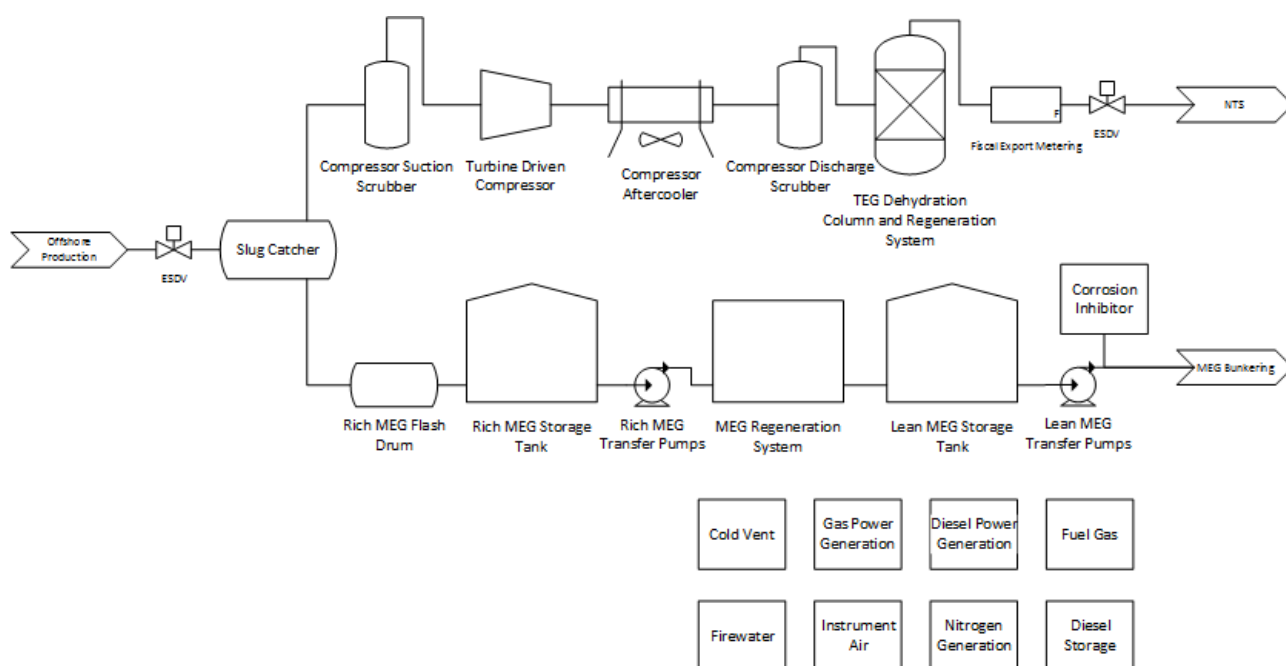
Figura 5.10 Schema tehnologică generală a GTP
