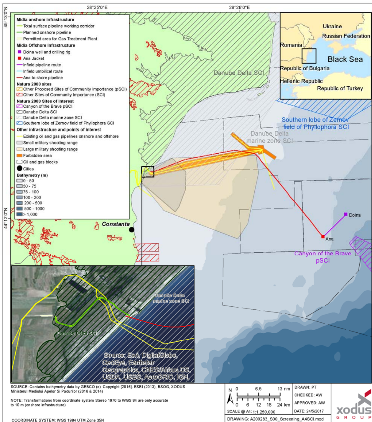
Figura 6.10 Situri de importanță comunitară (SCI) și propuse SCI
