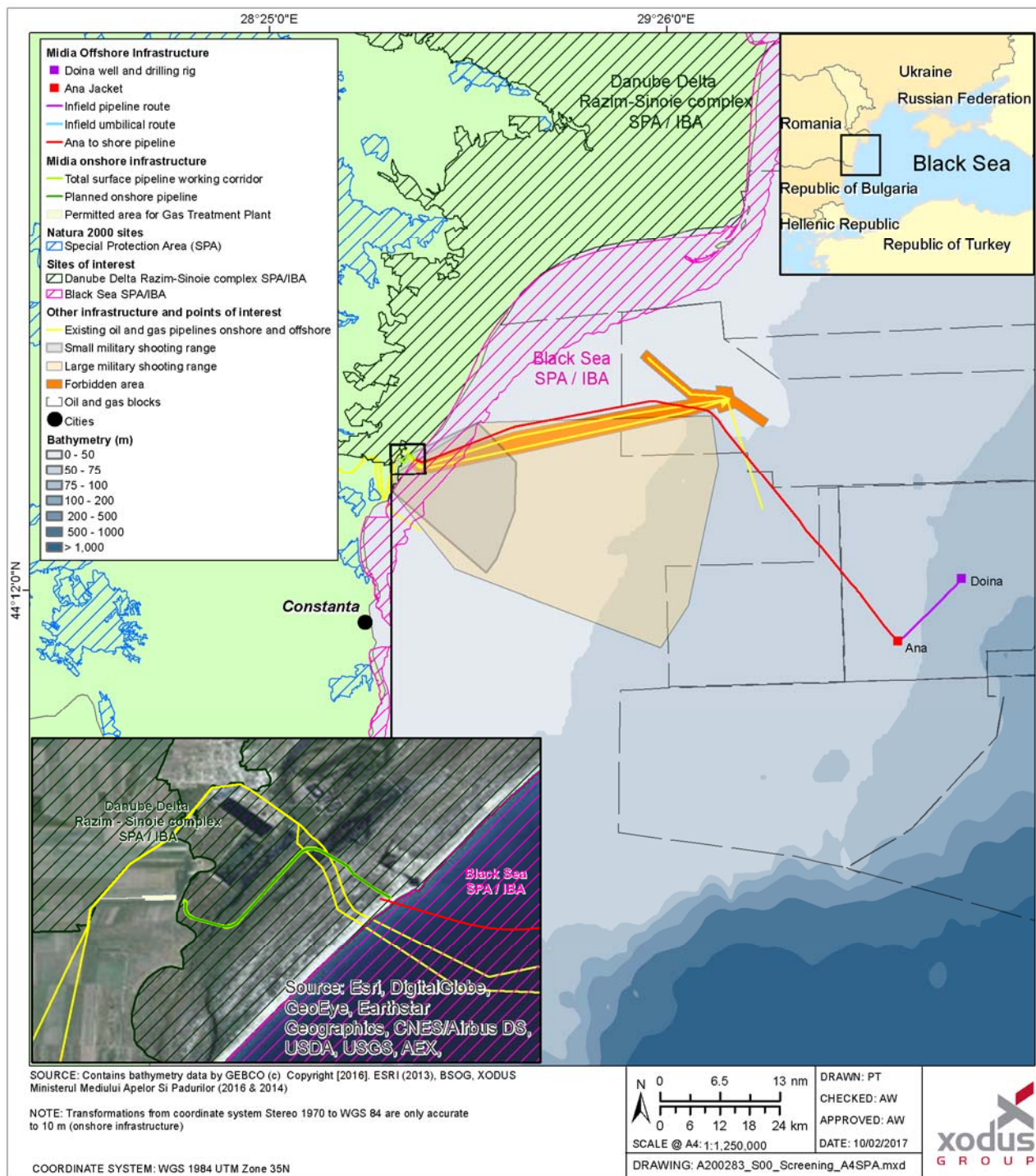
Figura 6.11 Zone de protecție specială (SPA) și zone importante pentru păsări (IBA)
