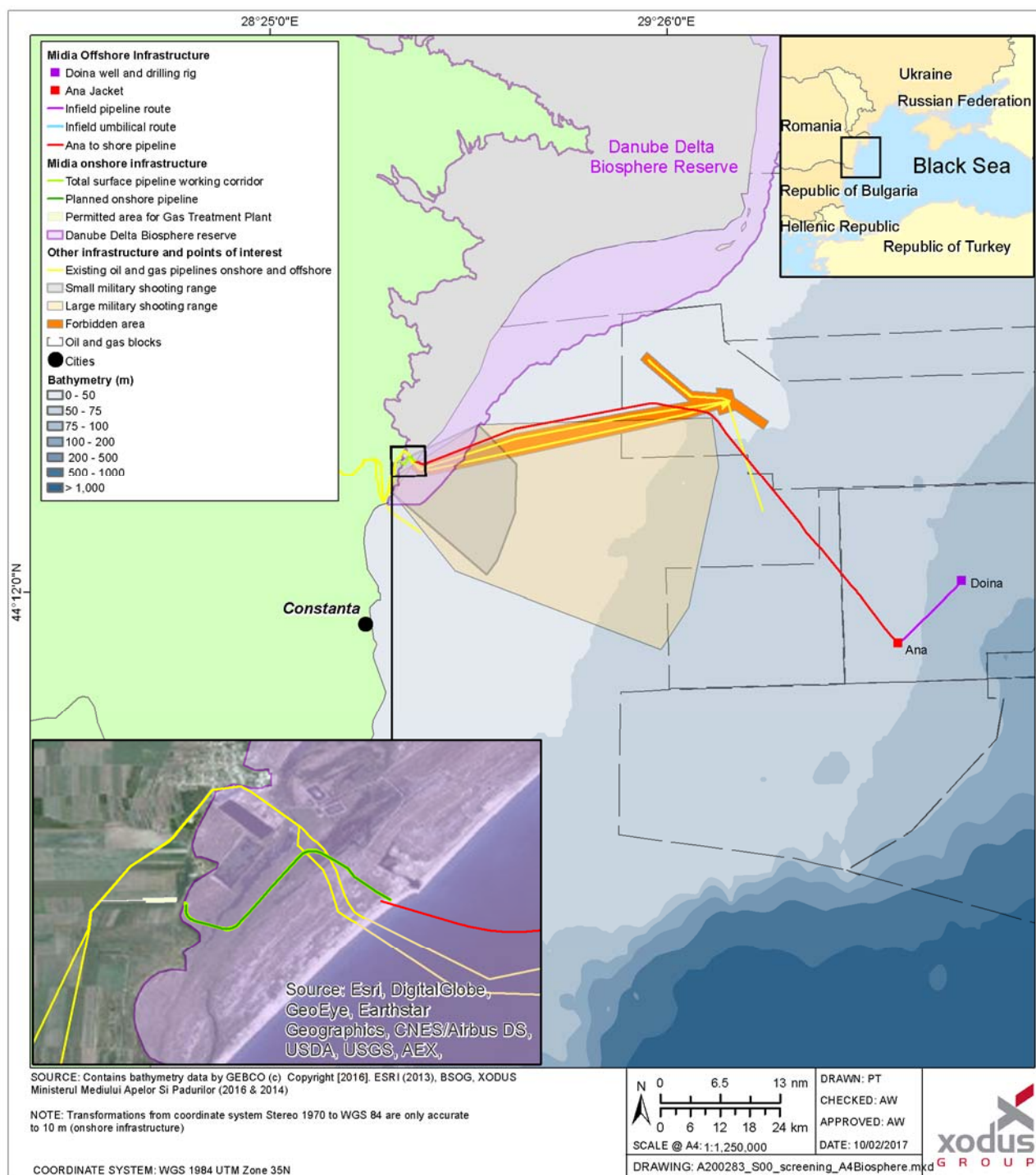
Figura 6.12 Rezervația biosferei din Delta Dunării
