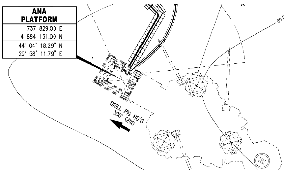
Figura 5.3 Orientarea platformei gurii de sondă Ana
