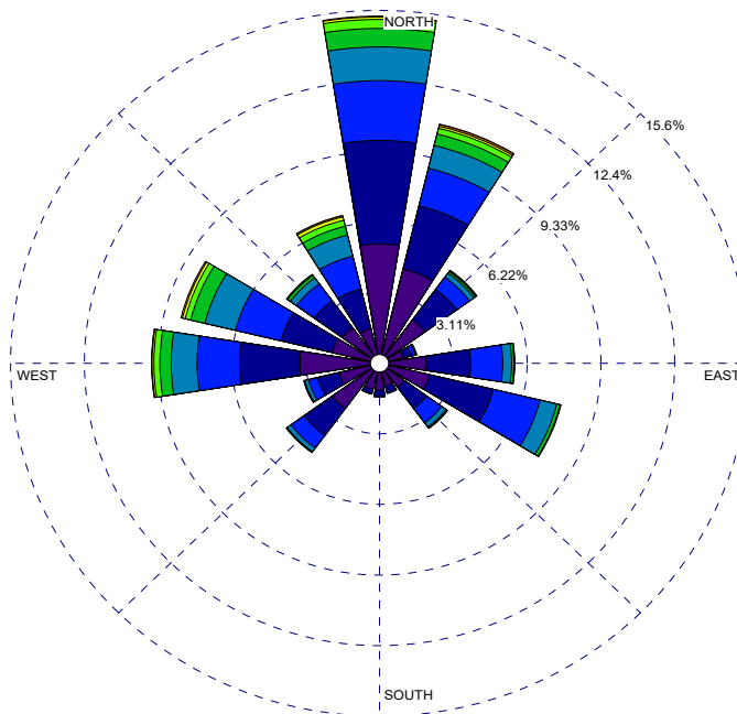
Figura 9.5 Roza vânturilor pentru datele meteorologice de la Constanța (2012 - 2016)
