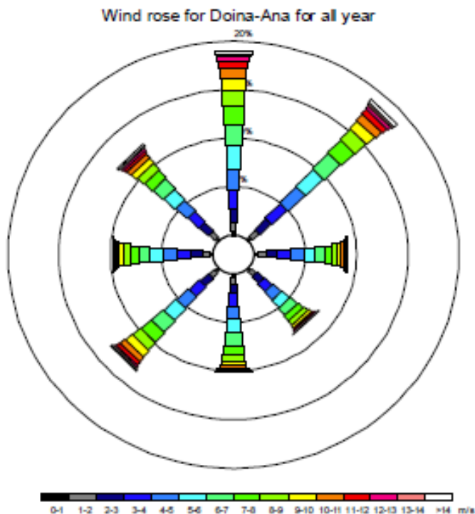
Figura 8.1 Roza vânturilor pentru Ana-Doina (BMT ARGOSS, 2017)
